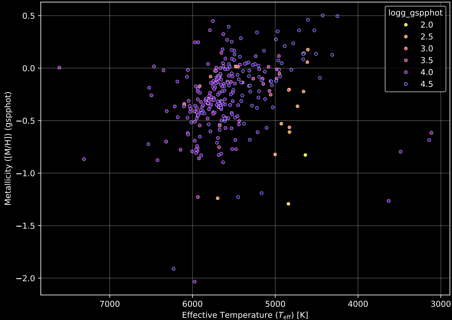
GALAH DR4 Field: [6888] Stellar Population Parameters (n= 288)
