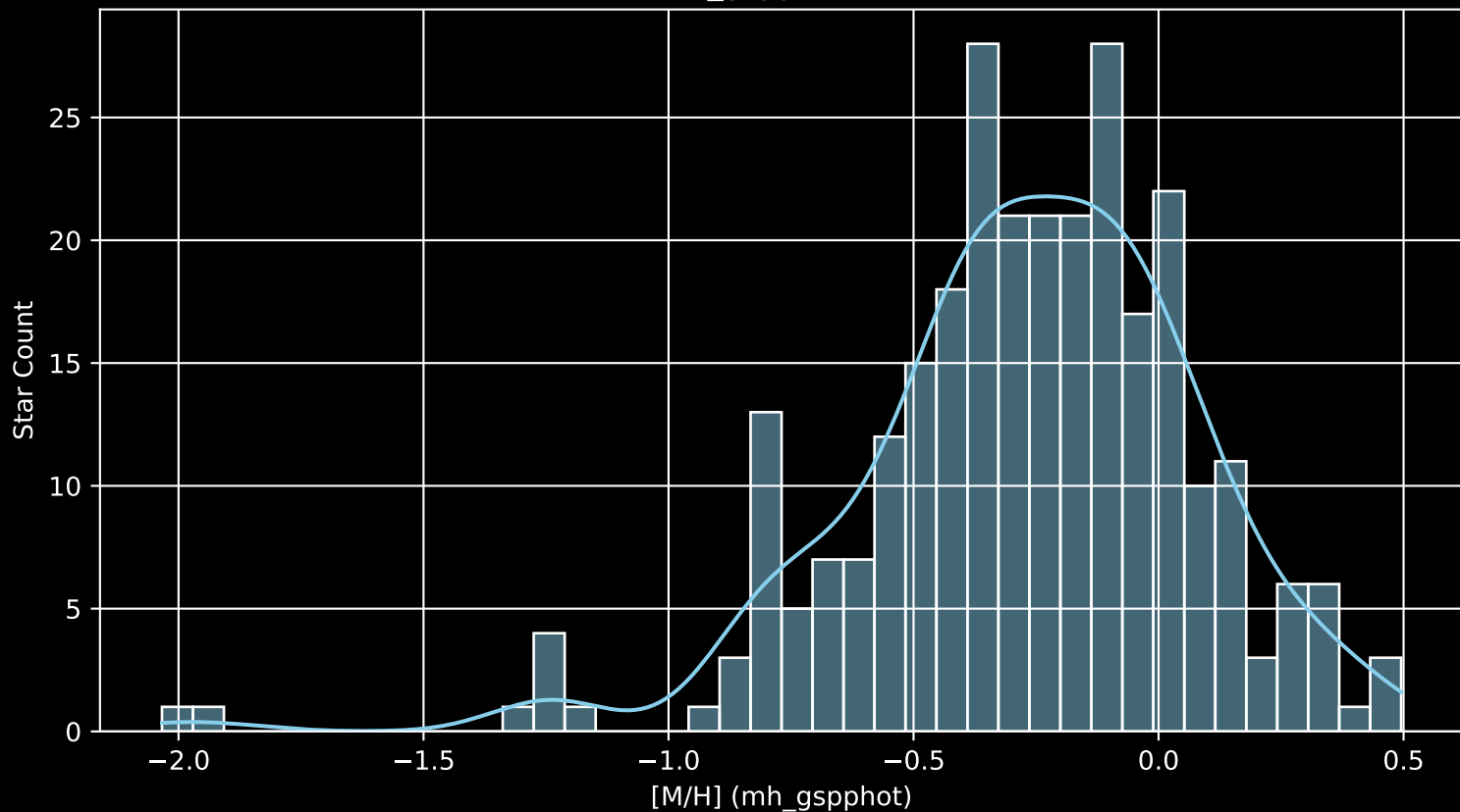
GALAH DR4 Field: [6888] [M/H] (mh_gspphot) (n= 287)
