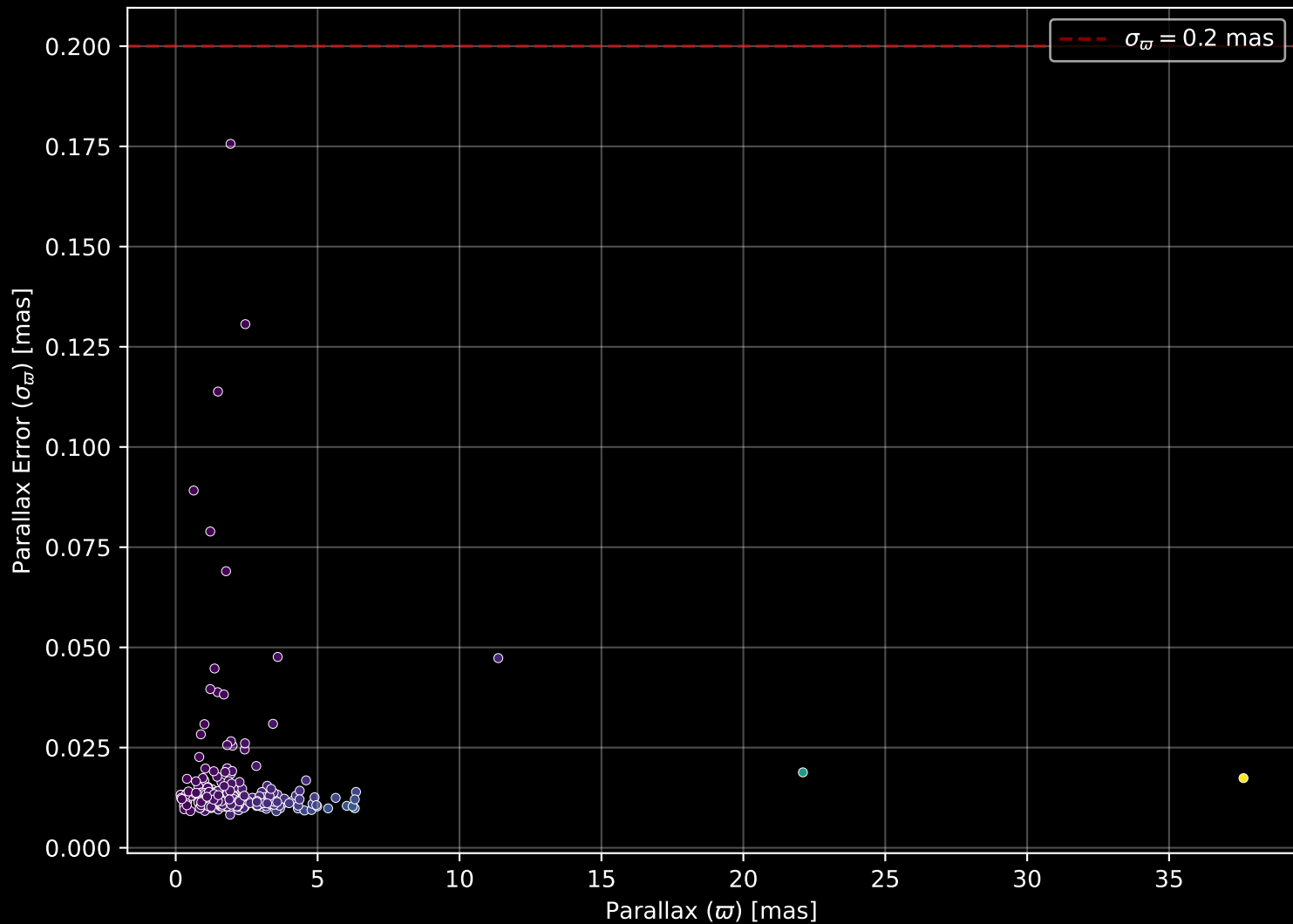
GALAH DR4 Field: [6888] Parallax Quality (n= 288)
